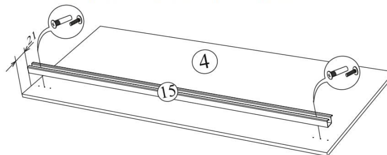
Modul de prindere al glisierii de placa superioară
