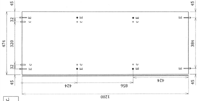
7. Intermediar Mare x 1buc. ( 1280 x 474 x 16 )
