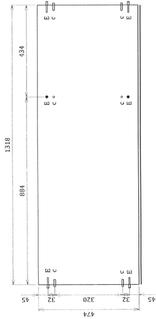
3. Polita Sus Dulap x 2buc. Z ( 1318 x 474 x 16 )
