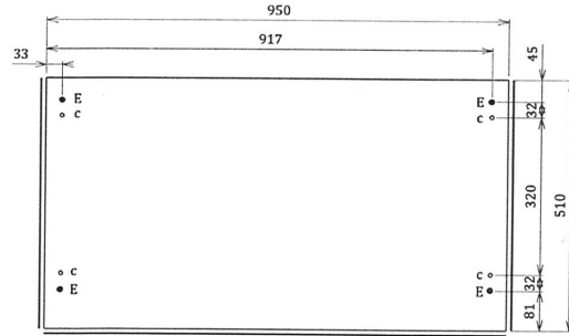
1. Capac Sus x 1buc. ( 950 x 510 x 16 )
