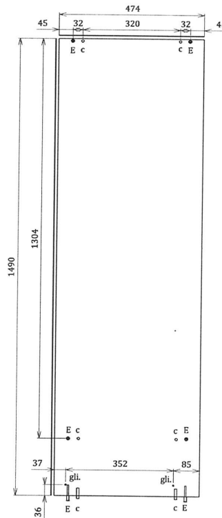
4. PL St Dulap x 1buc. ( 1490 x 474 x 16 )
