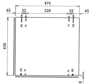
2. PL Suprapozabil x 2buc. ( St - Dr ) ( 430 x 474 x 16 )
