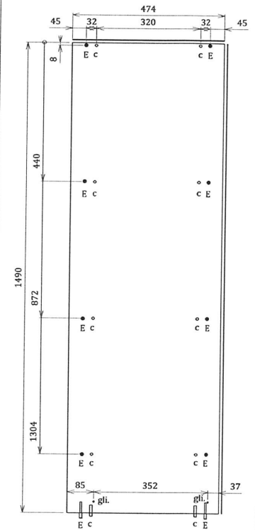
6. PL Dr Dulap x 1buc. ( 1490 x 474 x 16 )
