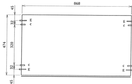
3. Polita Suprapozabil x 1buc. ( 868 x 474 x 16 )
